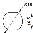
Шаблон для сверления двери шкафа и установки замка
