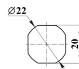
Шаблон для сверления двери шкафа и установки замка
