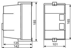
Рис.4.2 Габаритные и установочные размеры КМИ-22560.
