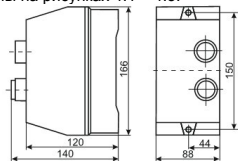
Рис.4.1 Габаритные и установочные размеры КМИ-10960 – КМИ-11860.
