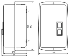
Рис.4.3 Габаритные и установочные размеры КМИ-34062 – КМИ- 49562.
