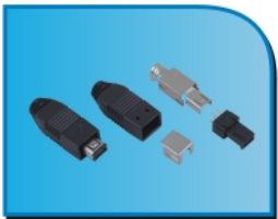
172 SERIES MINI USB-A MALE 4PIN SOLDER
