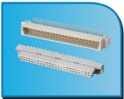
145 SERIES DIN41612 3B /4 TYPE(2ROWS)
