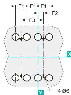
TEM7(E)-125-630 4P
