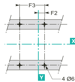
TEM7(E)-125-630 4P
