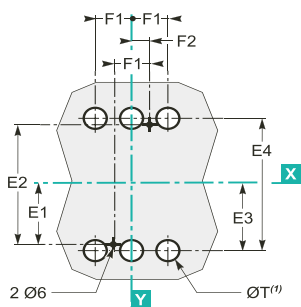
TEM7(E)-125/250 3P
