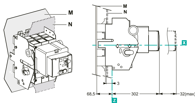
Монтаж моторного привода на выключателе выкатного исполнения
