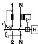
Схема подключения
