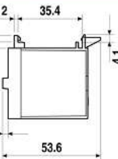
Адаптер 35 мм рейки (EN 60715) для реле типов 65.31.xxxx.xxx9
