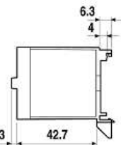
Адаптер 35 мм рейки (EN 60715) для реле типов 65.31.xxxx.xxx9
