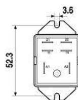
Фланцевый адаптер крепления для реле типов 65.31.xxxx.xxx9
