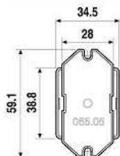
Фланцевый адаптер крепления для реле типов 65.31.xxxx.xxx9
