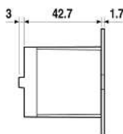
Фланцевый адаптер крепления для реле типов 65.31.xxxx.xxx9
