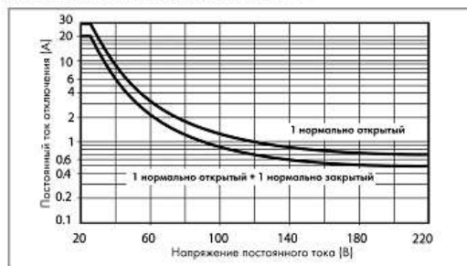
H 65 - Макс. отключающая способность DC1
