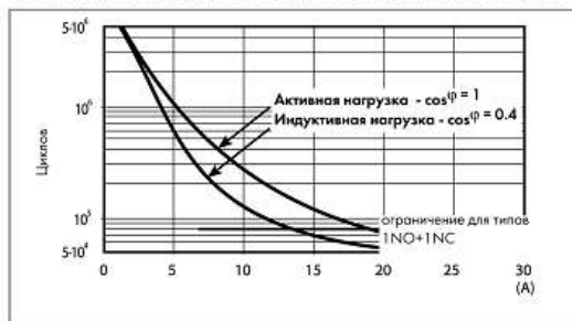
F 65 - Электрическая долговечность (AC) при номинальной нагрузке
